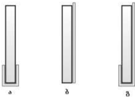
სურ. 21 – ლამელარის ფირფიტა გვერდიდან: ა. კიდეზე შემოფენილი ტყავით, ბ. უკან ტყავის საფენით, გ. ფირფიტის უკან და მის წინა ქვედა ნაწილზე ამოფენილი ტყავით.
